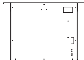
右側視圖
