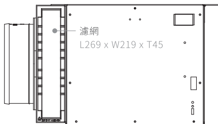
右側視圖
